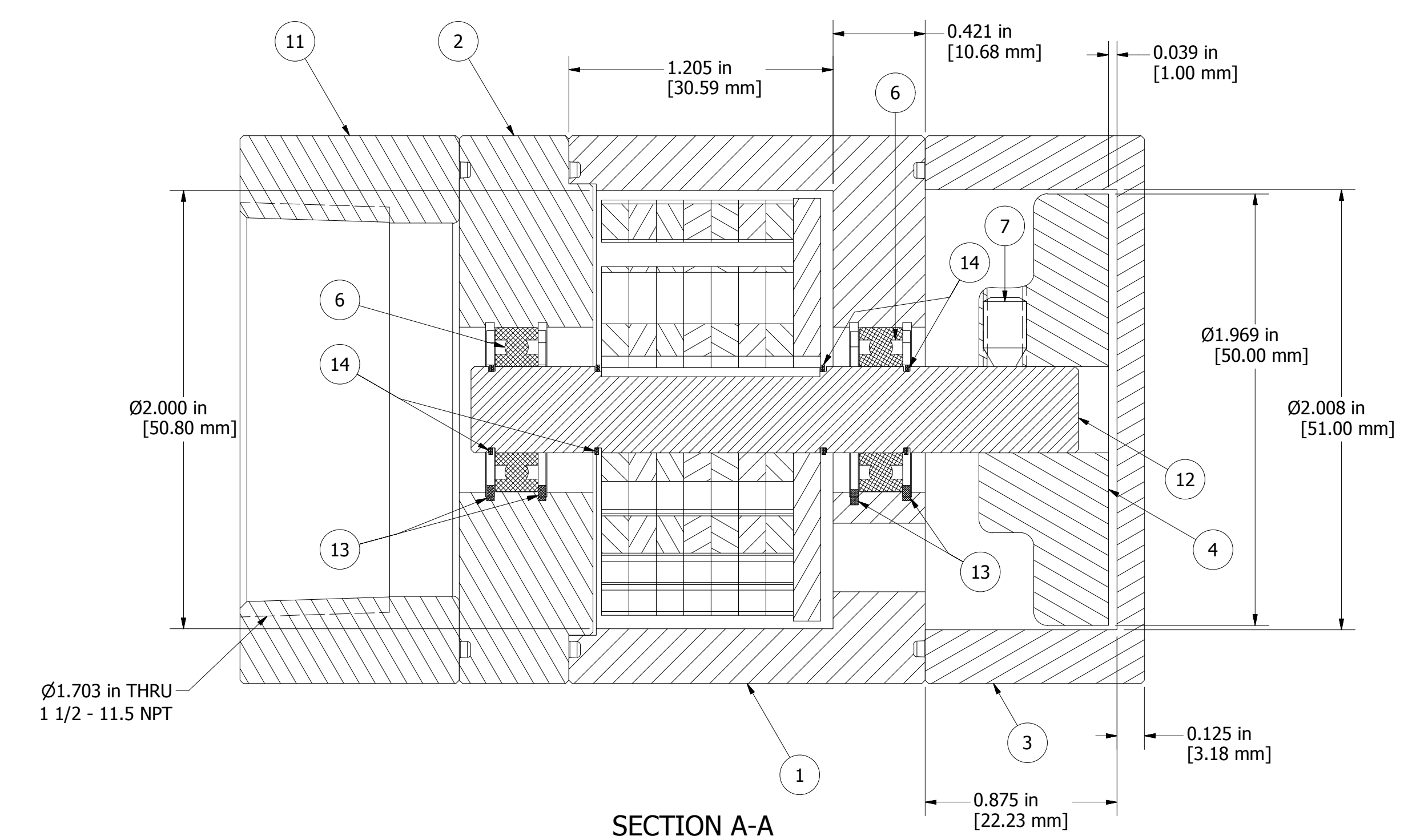
SECTION A-A SCALE 2 : 1
