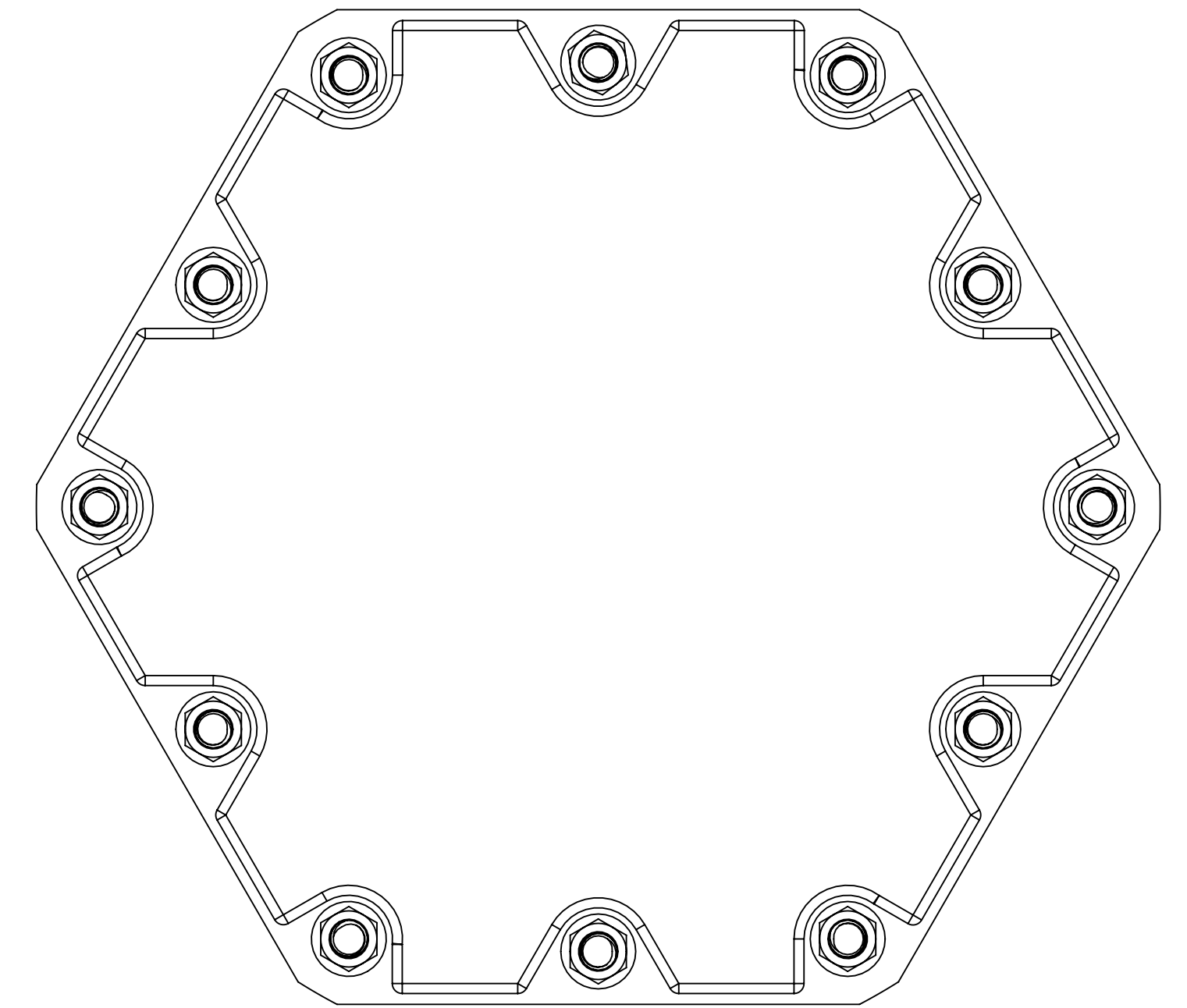
BACK VIEW SCALE: 1:1.5
